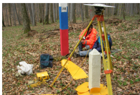
Meranie polygónového kameňa a vlícovacieho bodu metódou GPS.
